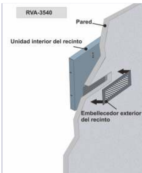
Rejilla de ventilación: Protección contra el fuego EI2-60
