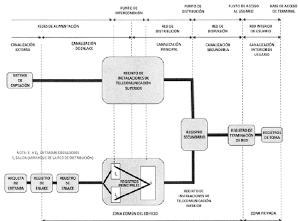
Apéndice 1: Esquema General de una ICT
