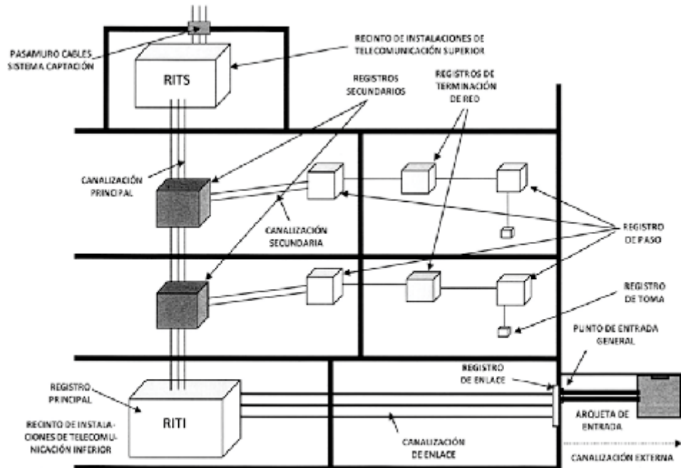
APENDICE 2: Esquema de canalizaciones para inmuebles de pisos
